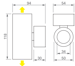
DIMENSIONI / DIMENSIONS
