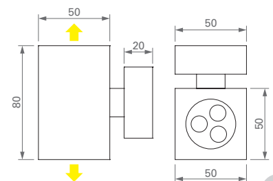
DIMENSIONI / DIMENSIONS
