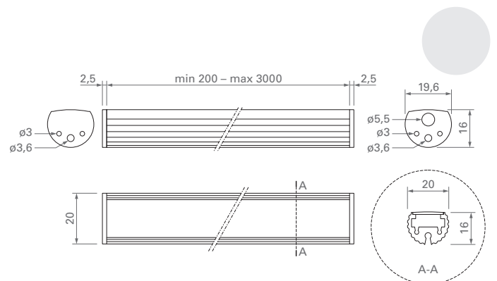
DIMENSIONI / DIMENSIONS
