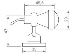
DIMENSIONI / DIMENSIONS
