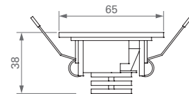
DIMENSIONI / DIMENSIONS
